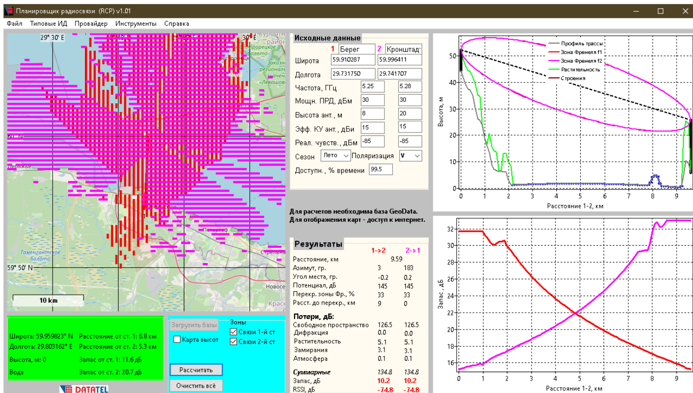
Рис. 13. Результаты расчета радиоканала и зон связи.
