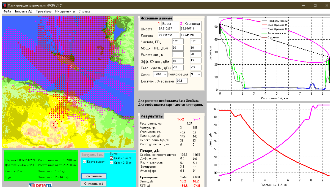
Рис. 14. Результаты расчета радиоканала и зон связи на карте высот.
